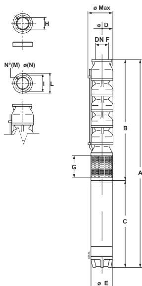
Overall dimensions and weights Dimensiones máximas y pesos Dimensioni di ingombro e pesi
