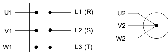
Conexão do quadro
