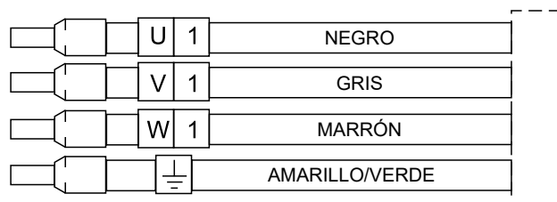
Identificación conductores cable electrobombas
