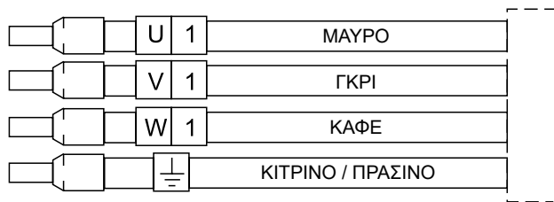
Αναγνώριση αγωγών καλωδίου ηλεκτρικών
