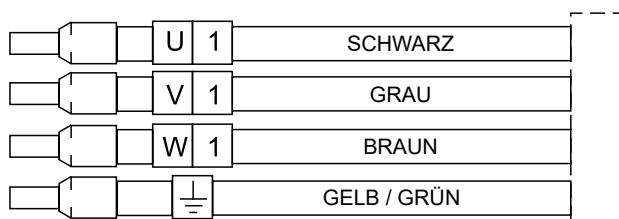
Identifizierung der Leiter der Elektropumpenkabel
