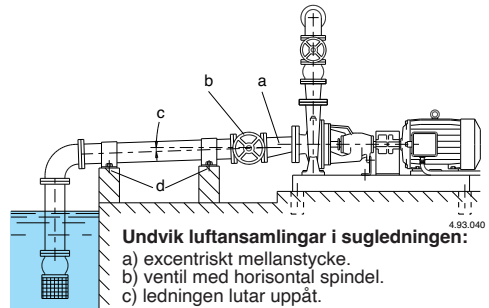
Bild 4 Anslutning av rörledningarna.
