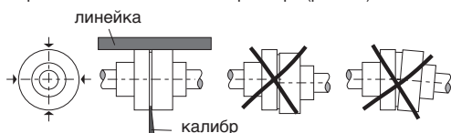
Рис. 6A Центровка соединения
