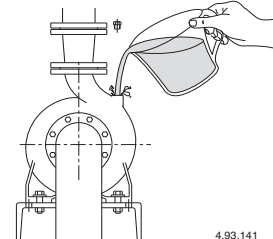
Fig. 8 Riempimento.
