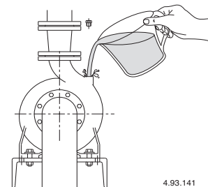
Abb. 8 Auffüllung.
