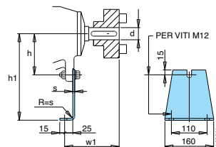
Fig. 7 Sostegno aggiunto del supporto.
