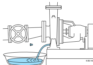
Рис. 9 Слив воды
