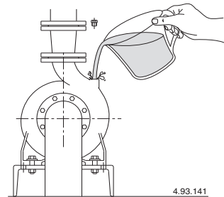
Bild 8 Fyllning.
