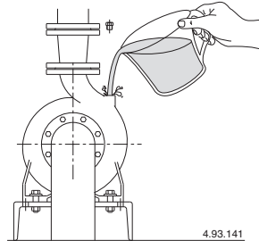
Fig. 8 Remplissage.
