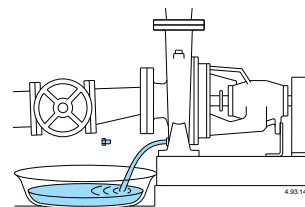
Fig. 9 Descarga.
