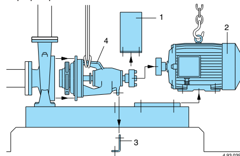
Fig. 10 Sequenza di smontaggio.
