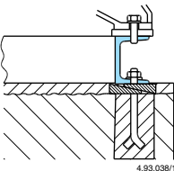
Fig. 3 Fundatie per gemonteerd zijn op een gelast staal-profiel grondplaat
