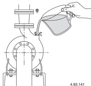
Fig. 3 Cebado.
