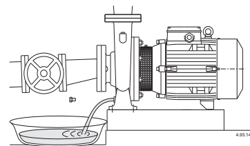
Σχ. 4 Αποστράγγιση
