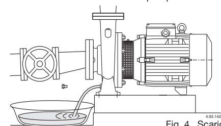
Fig. 4 Scarico.
