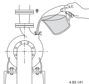
Рис. 3 Заполнение жидкостью
