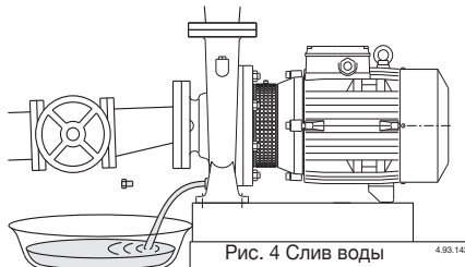
Рис. 4 Слив воды
