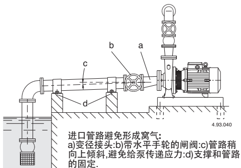
图2 管路连接
