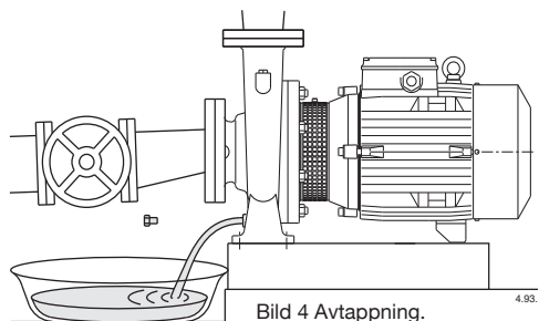
Bild 4 Avtappning.
