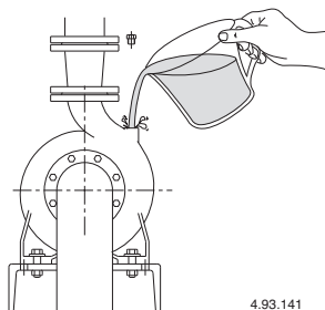
Abb. 3 Auffüllung.
