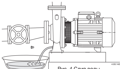
Рис. 4 Слив воды
