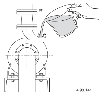
图.3 灌泵
