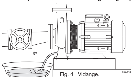
Fig. 4 Vidange.
