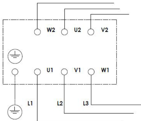
ABBILDUNG 11.1. Δ - Anschluss (dreieckig)
